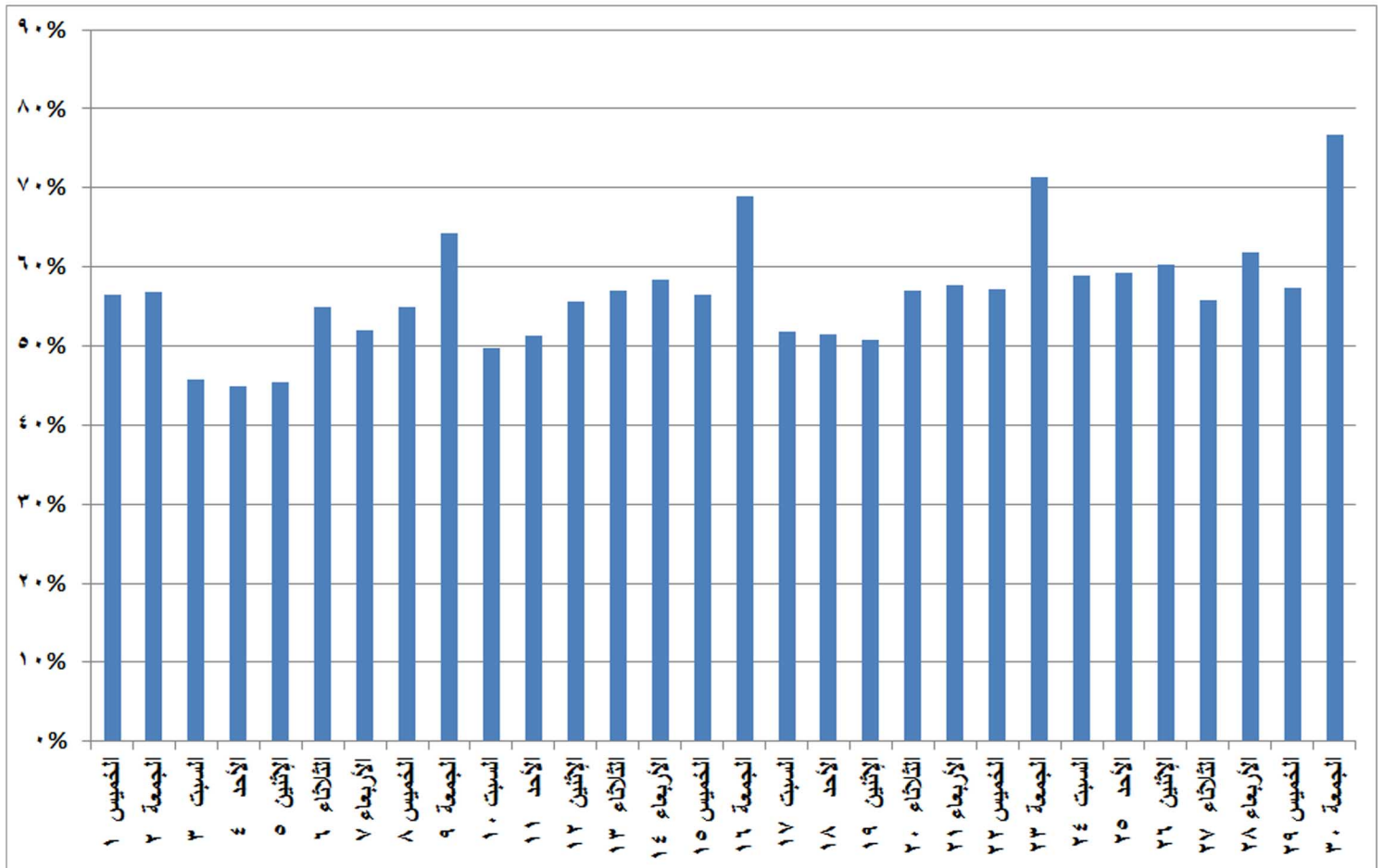
شكل (٢٨) نسب الفائض للحمل الاقصى المسجل يوميا خلال شهر نوفمبر ٢٠١٨
