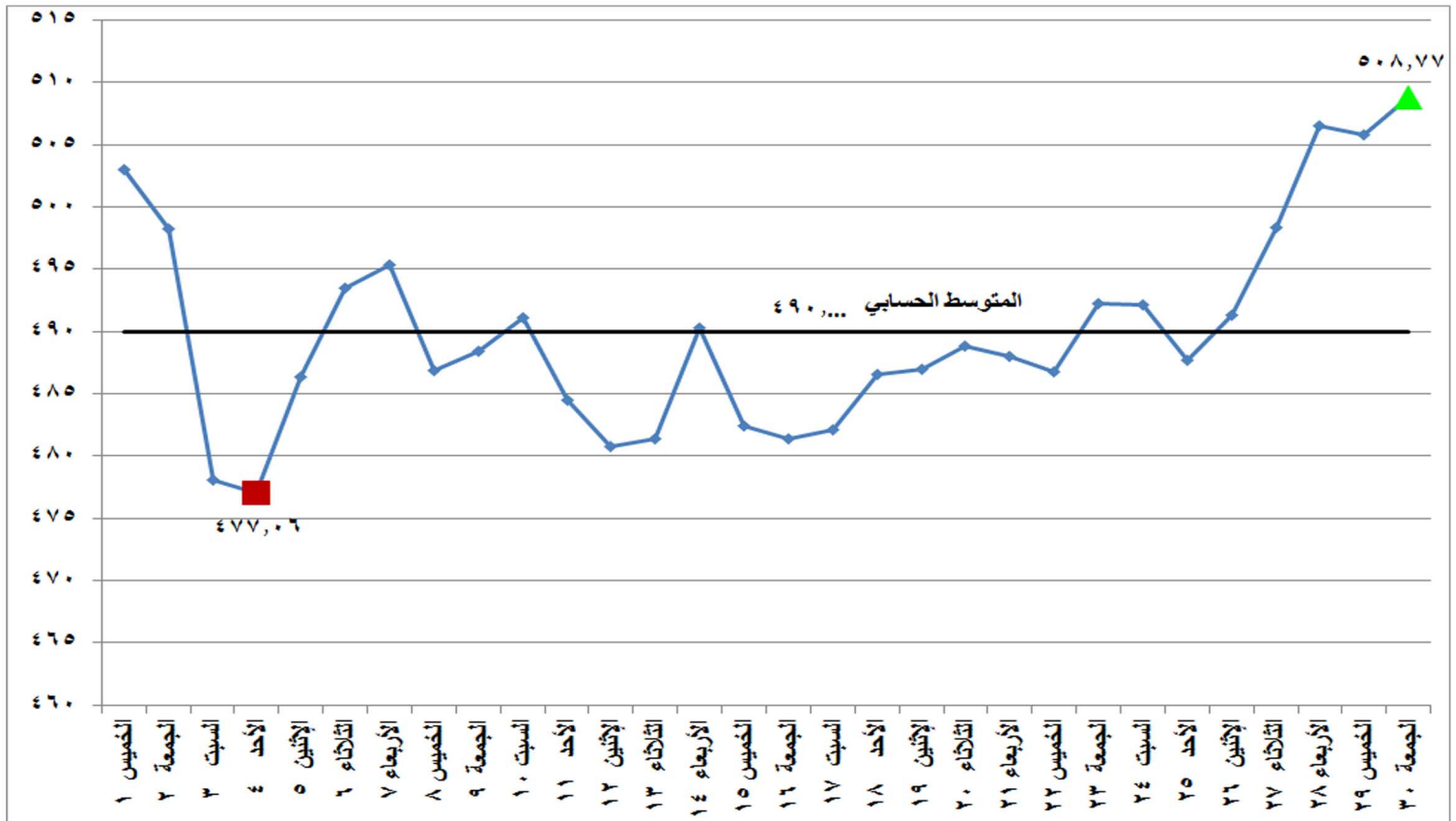
شكل (١٤) معامل انبعاثات غاز ثاني اكسيد الكربون المكافئ على مدى شهر نوفمبر ٢٠١٨
