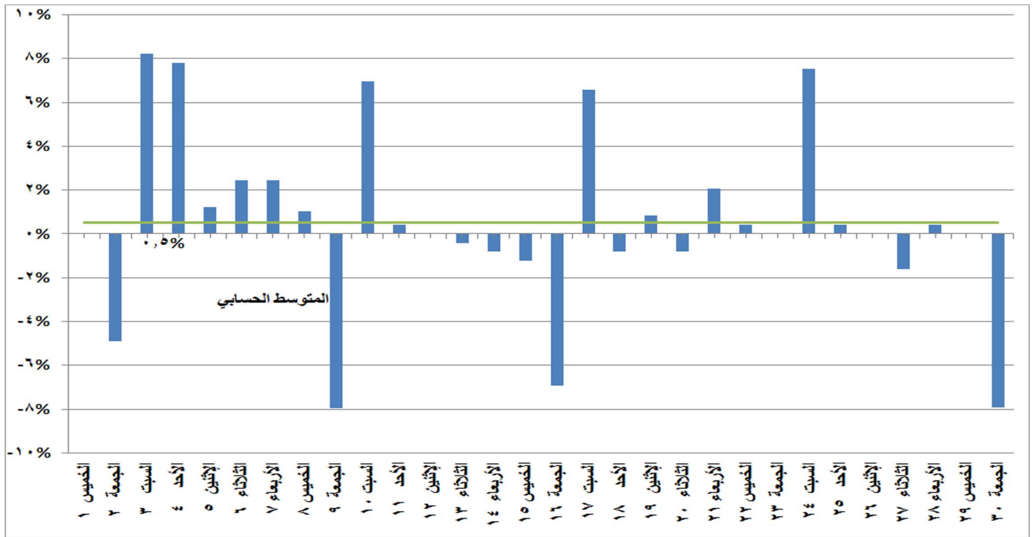
شكل (٩) النسب المئوية للتغير في الحمل الاقصى خلال شهر نوفمبر ٢٠١٨ مقارنة باليوم المماثل من العام الماضي
