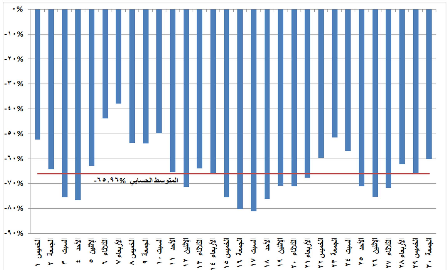
شكل (٢٠) نسب التغير في استخدام المازوت في إنتاج الطاقة الكهربائية خلال شهر نوفمبر ٢٠١٨ مقارنة بالشهر المماثل من العام السابق
