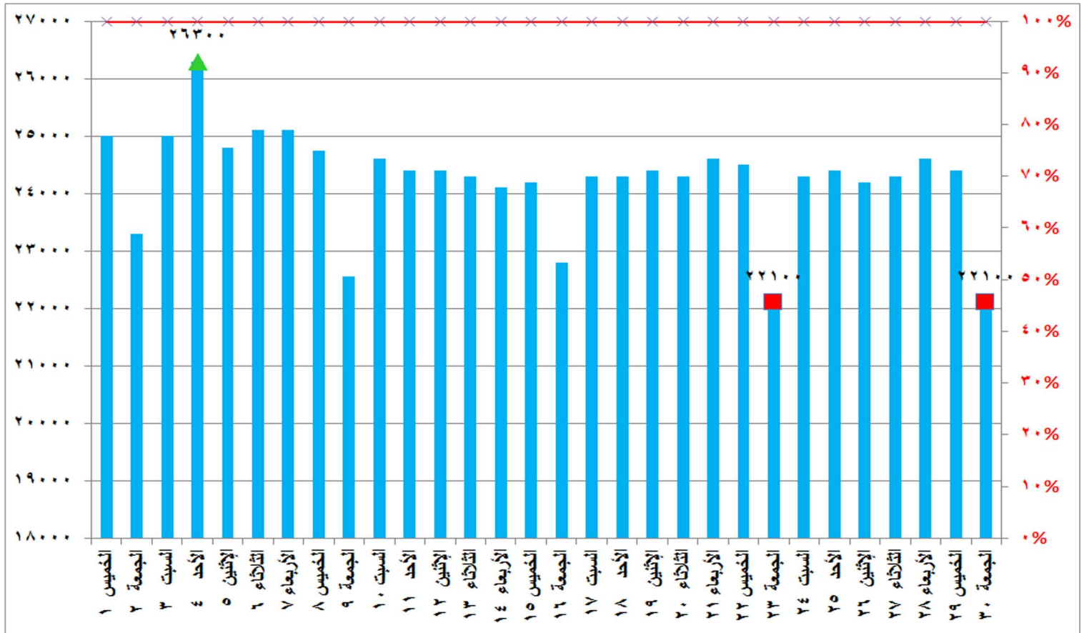
شكل (٥) قدرات الانتاج المتاحة ونسبتها للحمل الأقصى خلال شهر نوفمبر ٢٠١٨
