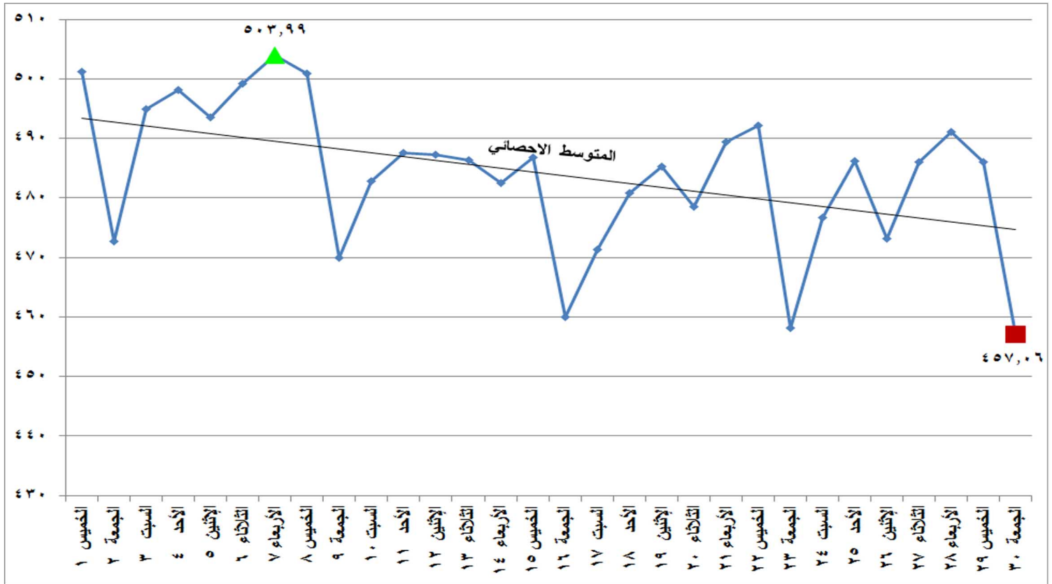
شكل (١٥) إجمالي الطاقة الكهربائية المنتجة من كل المصادر الأولية خلال شهر نوفمبر ٢٠١٨
