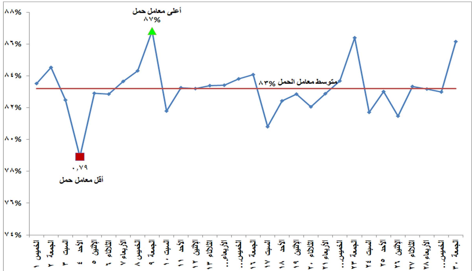
شكل (١٢) إجمالي معامل الحمل لوحدات الانتاج خلال شهر نوفمبر ٢٠١٨
