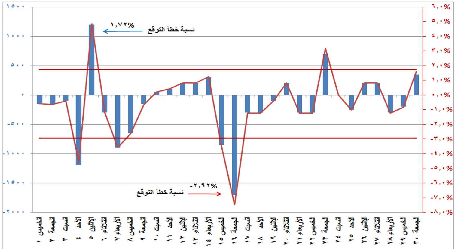
شكل (١٠) الفرق بين الحمل الأقصى المتوقع والمسجل فعليا ونسبة الفرق إلى الحمل المسجل فعليا خلال شهر نوفمبر ٢٠١٨
