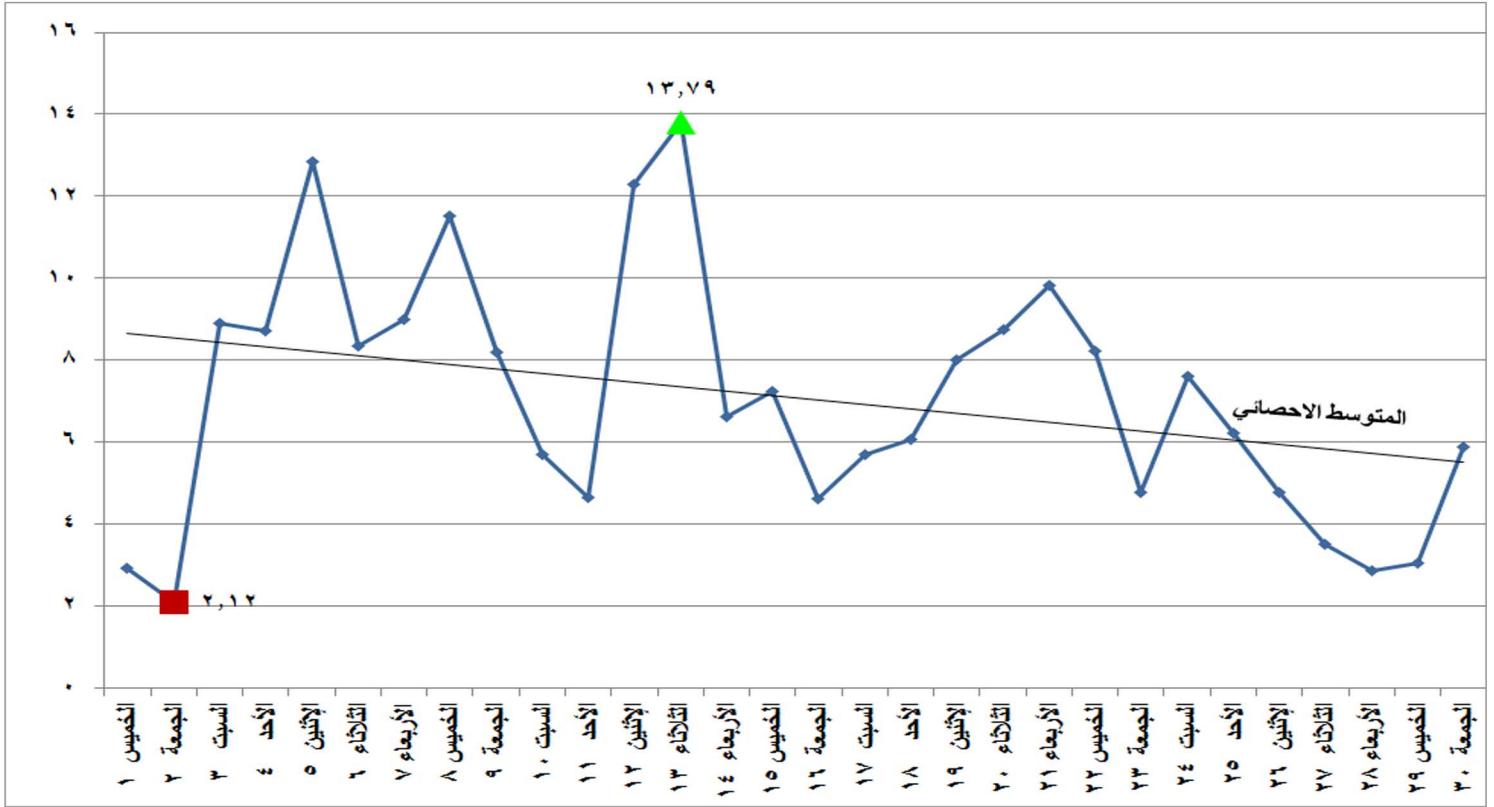
شكل (٢٥) الطاقة الكهربائية المنتجة من الرياح والشمس خلال شهر نوفمبر ٢٠١٨
