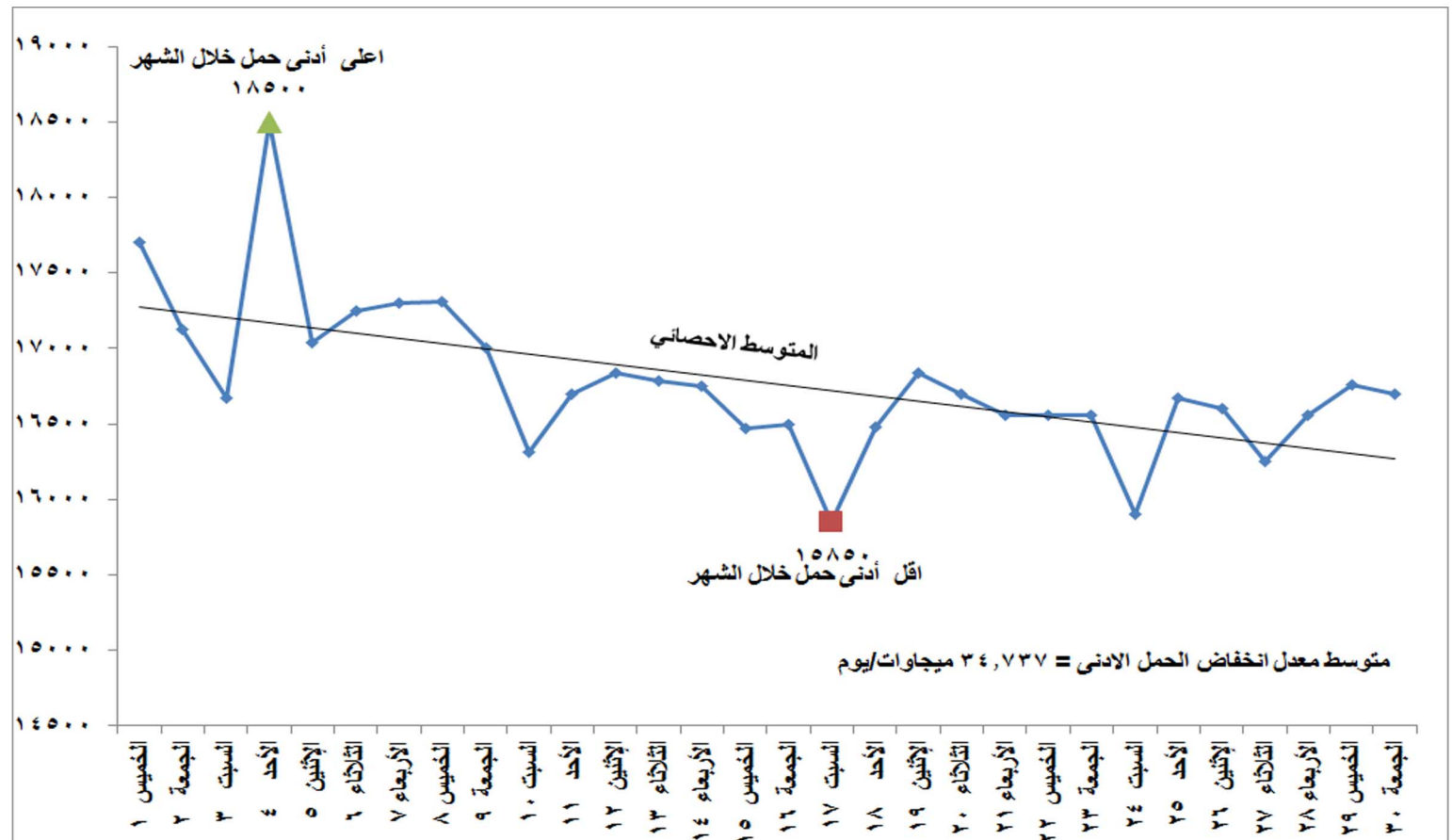
شكل (٢) تطور الحمل الادنى اليومي خلال شهر نوفمبر ٢٠١٨
