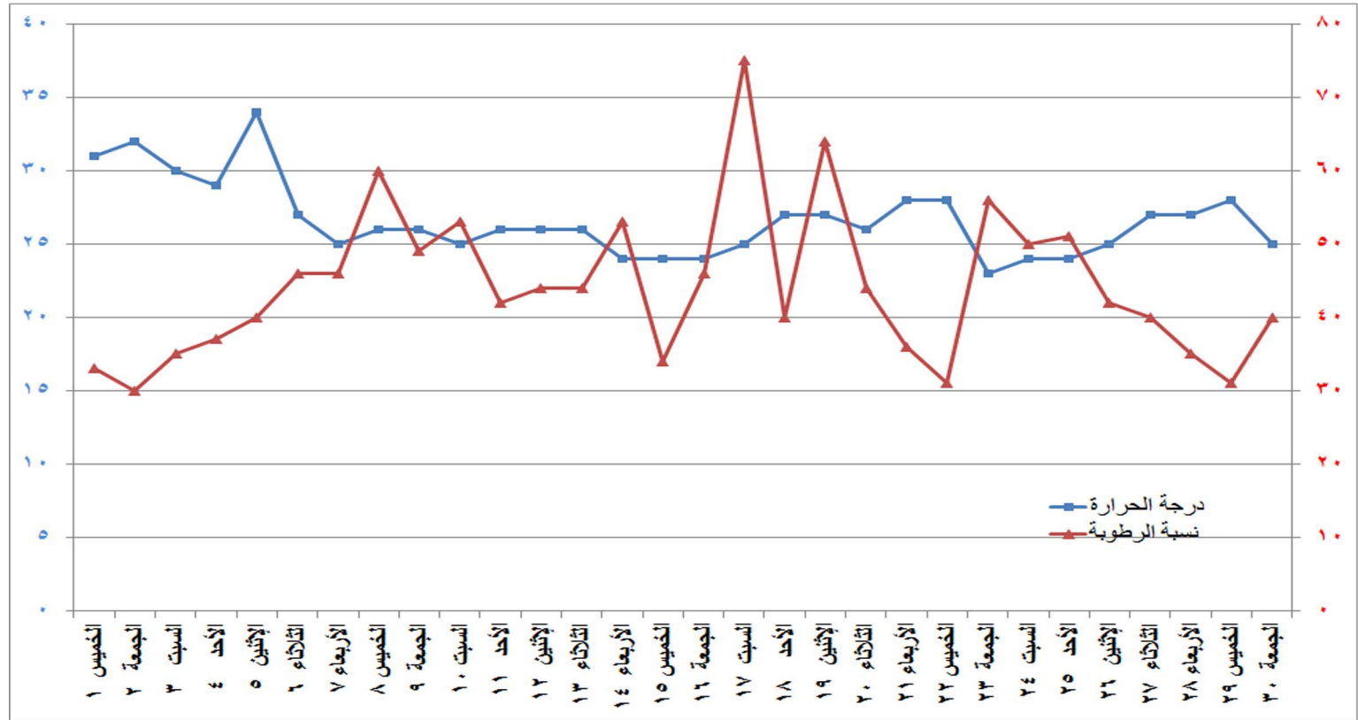
شكل (١١) التغيير في درجة الحرارة والرطوبة النسبية خلال شهر نوفمبر ٢٠١٨
