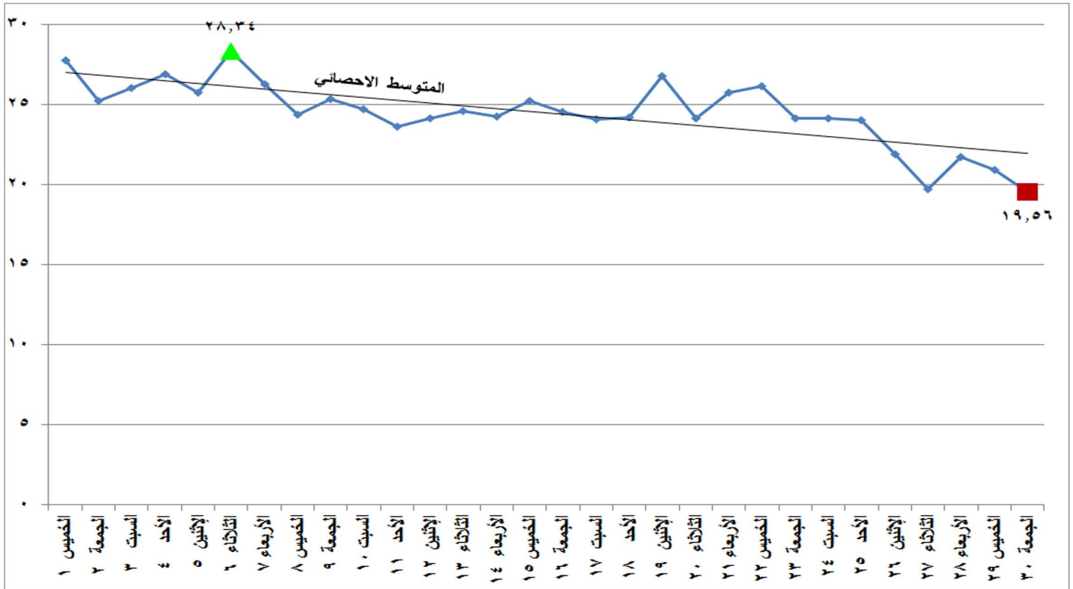
شكل (٢٣) الطاقة الكهربائية المنتجة من المصادر المائية خلال شهر نوفمبر ٢٠١٨
