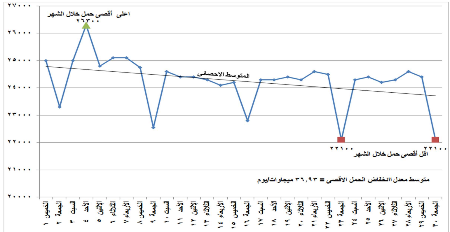
شكل (١) تطور الحمل الاقصى اليومي خلال شهر نوفمبر ٢٠١٨
