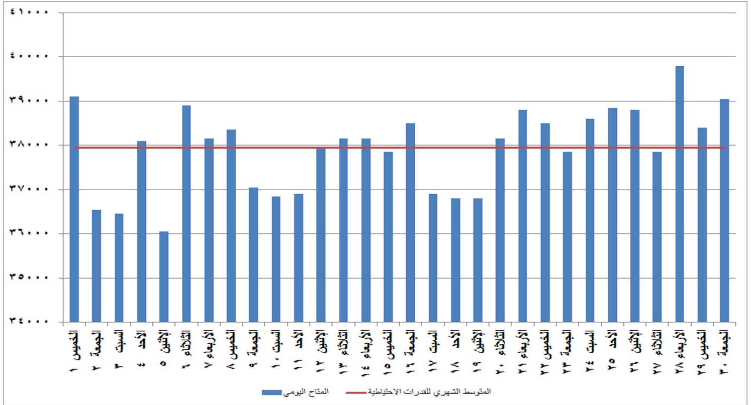
شكل (٢٧) القدرات المتاحة يوميا والمتوسط الشهري للقدرة الاحتياطية خلال شهر نوفمبر ٢٠١٨
